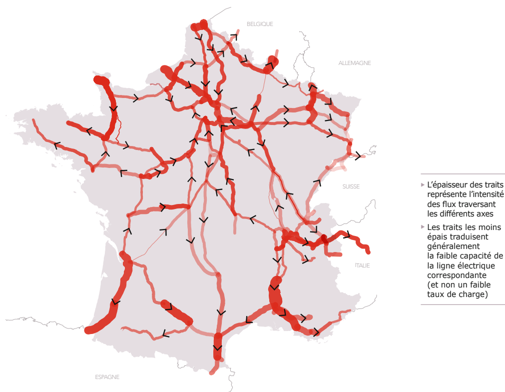
Figure 2. Illustration des flux sur le réseau de grand transport et les réseaux régionaux
