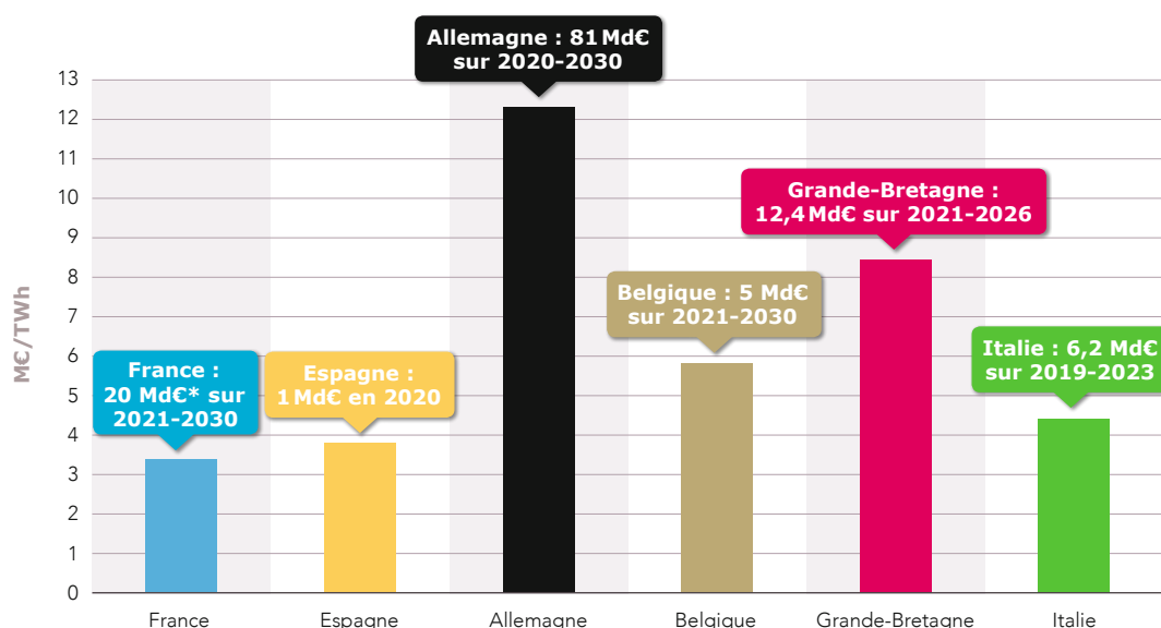
Figure 31. Investissements dans le réseau de transport d'électricité rapportés à la production électrique annuelle
