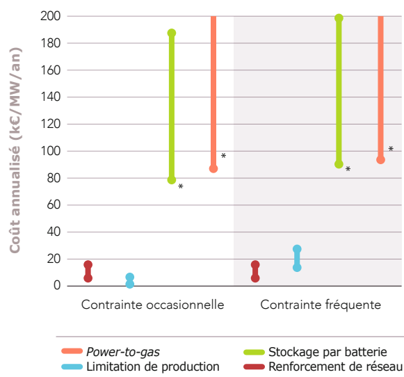
Figure 34. Comparaison économique de différentes solutions pour gérer les contraintes sur le réseau de transport (hypothèses de coûts 2018)
