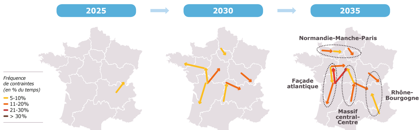
Figure 15. Projection des principales contraintes sur le réseau de grand transport en l'absence d'adaptation du réseau – scénario du projet de PPE et hypothèses de référence du SDDR
